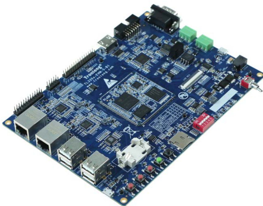
图 3 评估板斜视图
