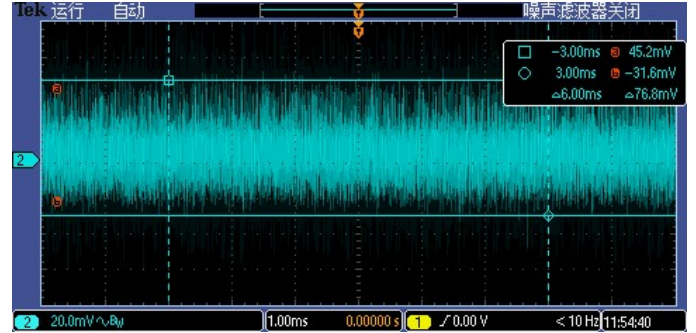
纹波波形图 4
